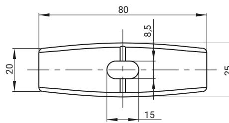
Ярмо 80 4.411.004
