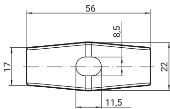
Ярмо 56 4.411.003
