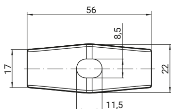
Jarzmo 56 4.411.003
