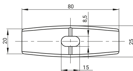
Jarzmo 80 4.411.004
