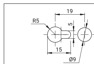
Otwory montażowe
