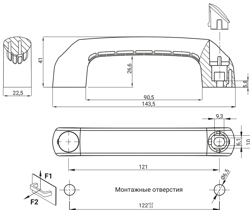
Ручка РА 4.444.002
