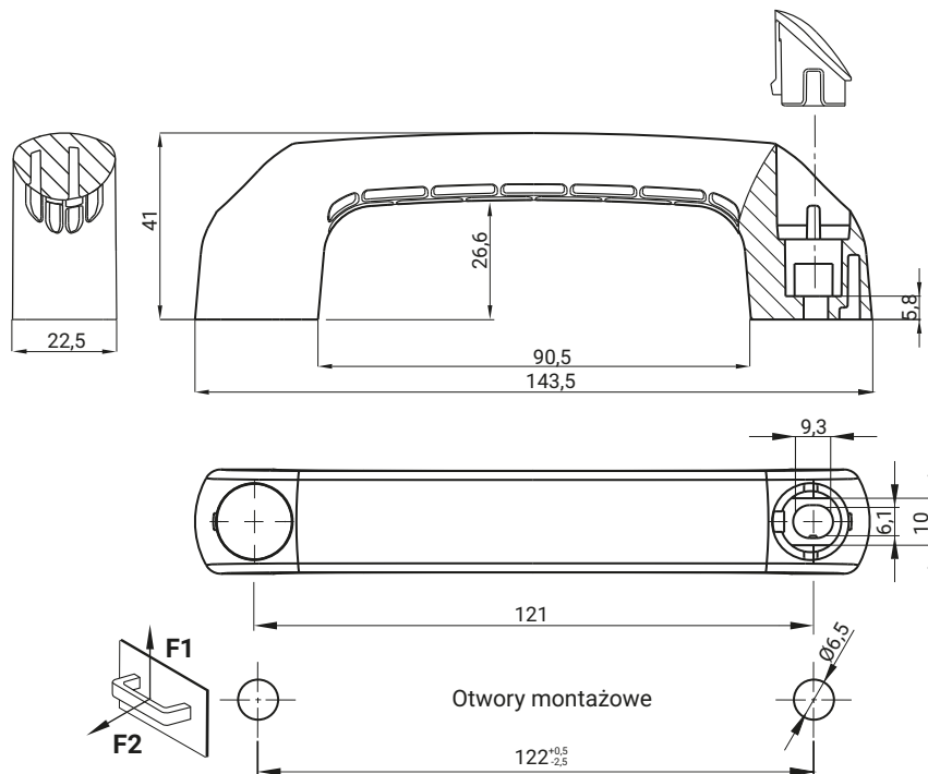
Uchwyt PA 4.444.002
