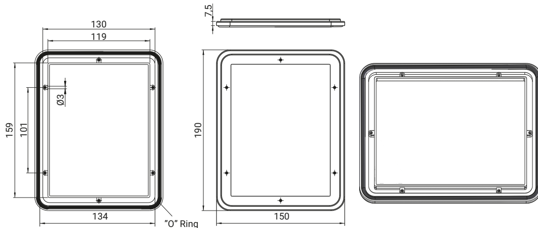
ОКОШКО 151 x 190
