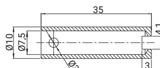
KLUCZYK 4.KDZN.002.06
