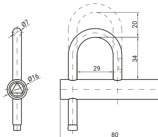
KŁÓDKA 4.KD.001
