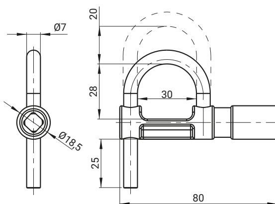
KŁÓDKA ZATRZASKOWA 4.KDZN.002
