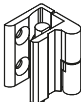
Zawias prawy
