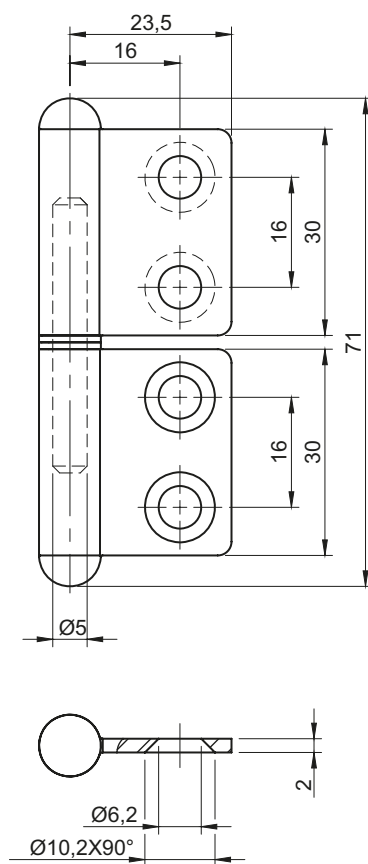
ZAWIAS LEWY 3.ST127.003SN - B
