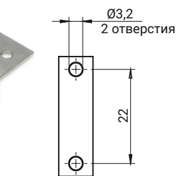
Монтажное отверстие
