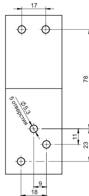
Монтажные отверстия
