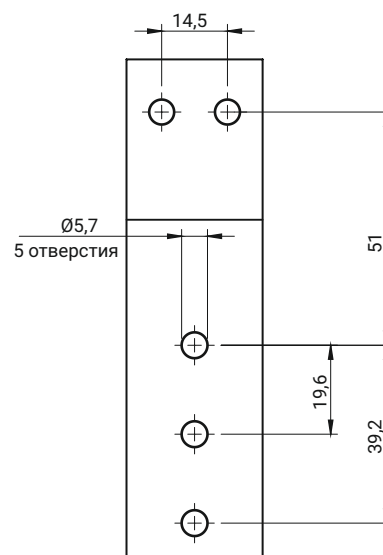
Монтажные отверстия
