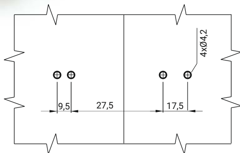
Otwory montażowe
