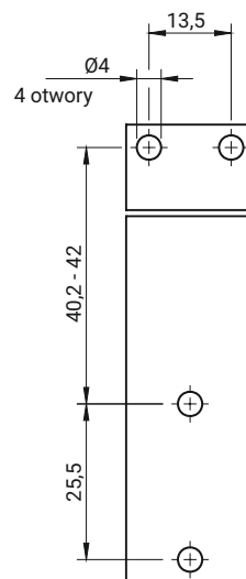
Otwór montażowy
