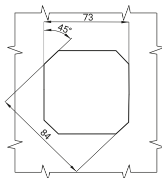
Otwór montażowy
