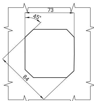
Otwór montażowy
