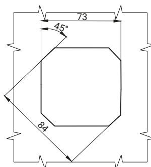
Otwór montażowy
