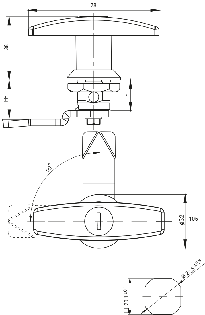
Otwór montażowy
