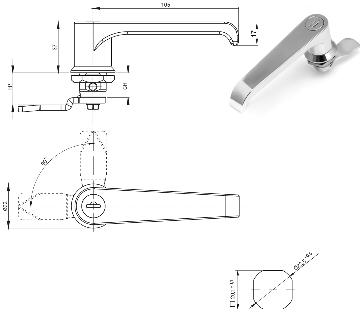
Otwór montażowy
