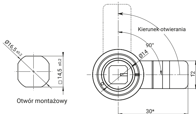
Zamek w wersji lewej
