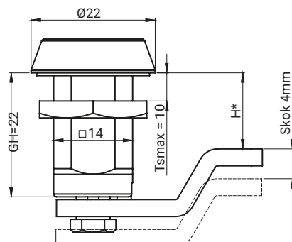
Wersja zamka A
