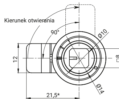
Zamek w wersji prawej
