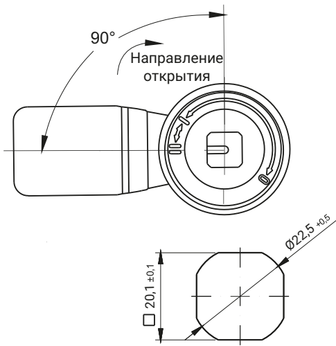
Монтажное отверстие
