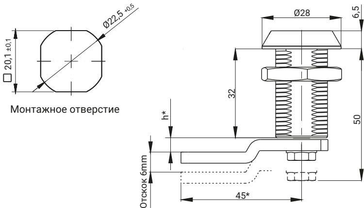
Версия замка А
