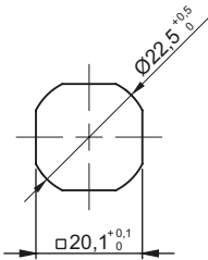
Монтажное отверстие
