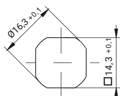
Монтажное отверстие
