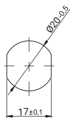
Otwór montażowy
