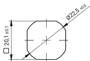
Монтажное отверстие
