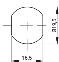
Otwór montażowy
