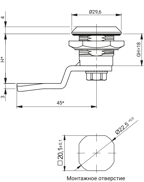
M22-8 - Тип замка с уплотнением PUR
