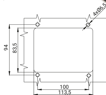
Otwór montażowy
