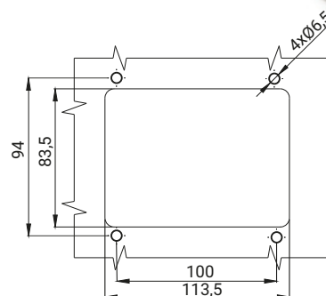
Otwór montażowy
