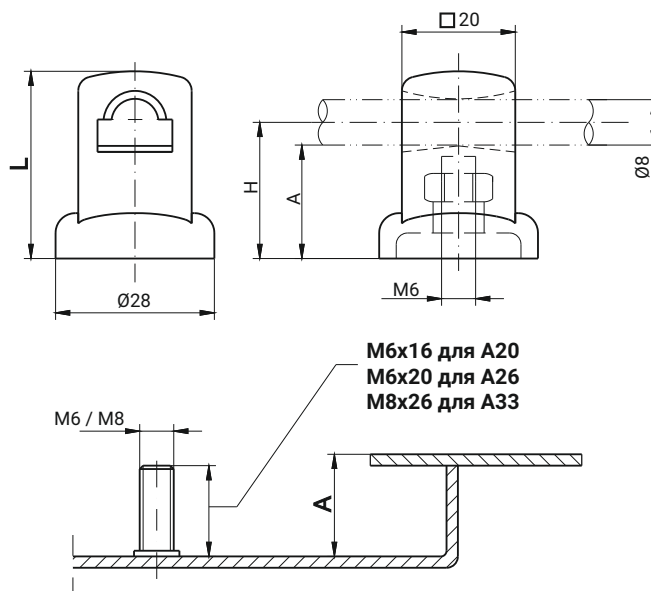
НАПРАВЛЯЮЩАЯ RW 1C.906.013
