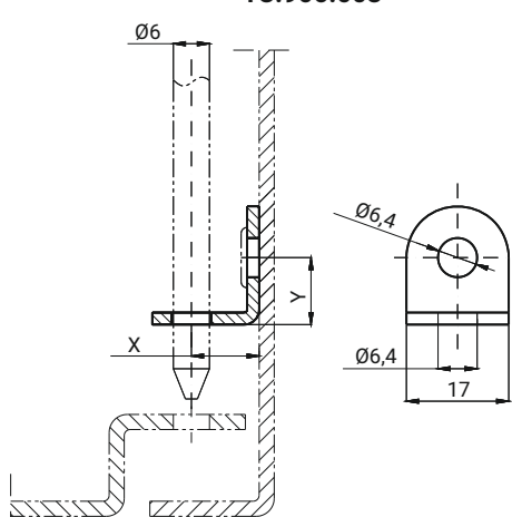
НАПРАВЛЯЮЩАЯ Ø6 - L 1C.906.003
