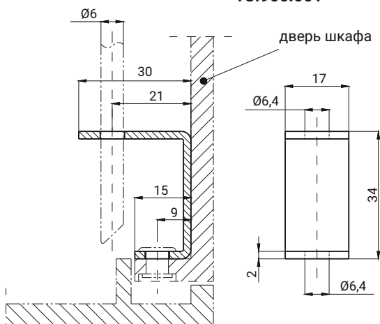
НАПРАВЛЯЮЩАЯ Ø6 - U 1C.906.001
