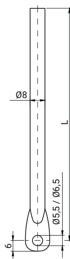
ТЯГА С ПЛОСКИМ КОНЦОМ (P48/U L)
