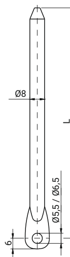
ТЯГА СО КОНУСНЫМ КОНЦОМ (P28/U L)
