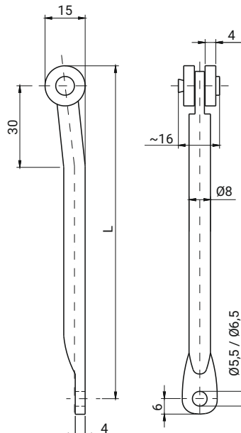
ТЯГА С РОЛИКАМИ (P38 L)
