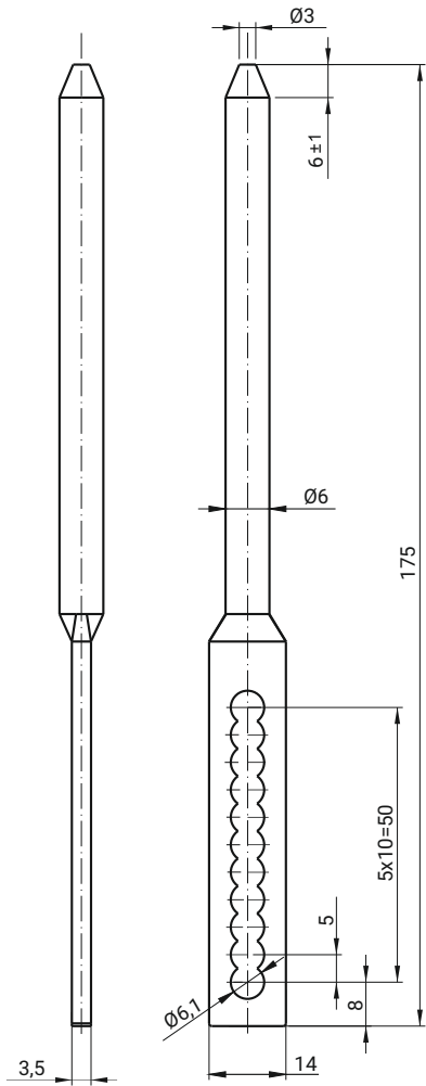
ТЯГА С КОНУСНЫМ КОНЦОМ РЕГУЛИРОВАННАЯ (PR28L)
