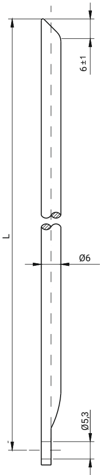
ТЯГА С СРЕЗАННЫМ КОНЦОМ (P16L)
