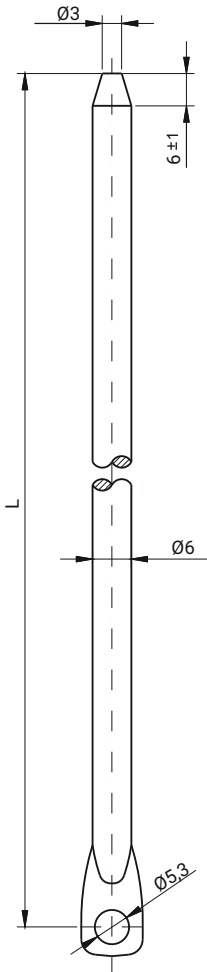
ТЯГА С КОНУСНЫМ КОНЦОМ (P26L)
