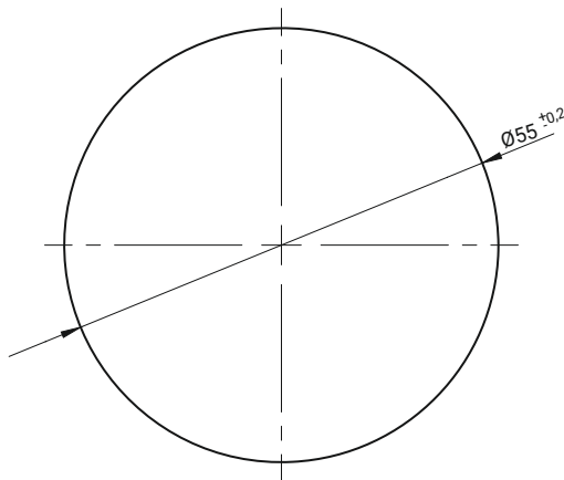
Монтажное отверстие 1C.916.002 i 1C.916.003
