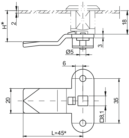
ЯЗЫК 3-пкт (с ограничителем и элементом для защиты)
