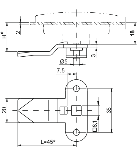
ЯЗЫК 3-пкт (с ограничителем и элементом для защиты под накладку)
