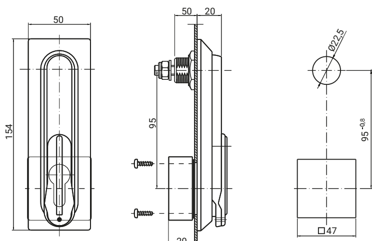
Kształt i wymiar otworów do osadzenia zamka
