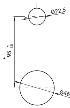
Otwór montażowy
