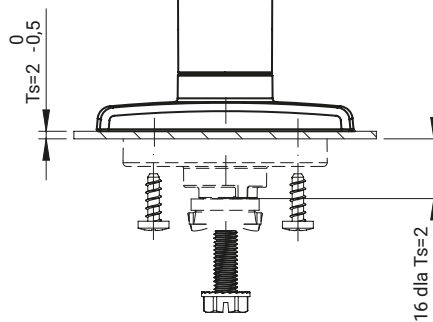
RW525.M (zamek pod mechanizm zębany)
