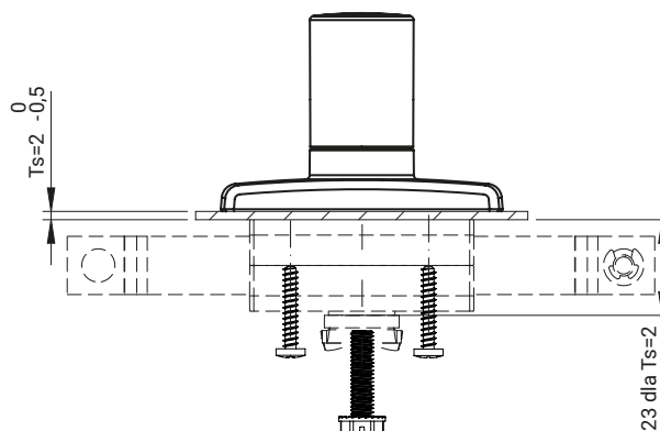
RW525.M (zamek pod mechanizm zębany)
