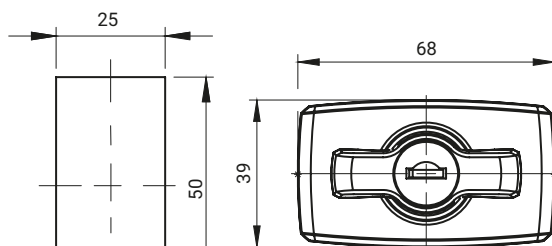
Otwór montażowy
