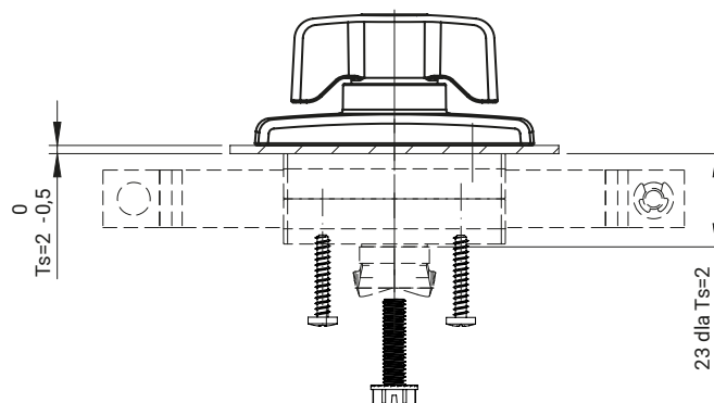
RW505.M (zamek pod mechanizm zębaty)
