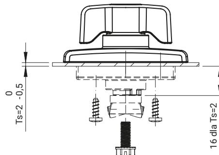
RW505.N (zamek pod nakładkę)
