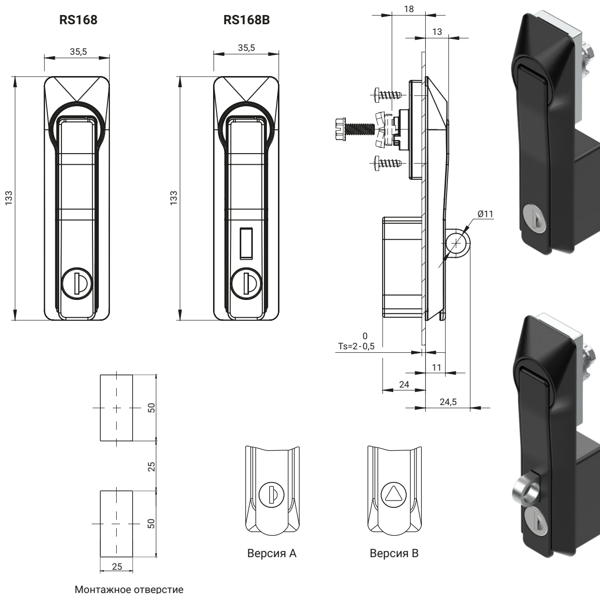
Монтажное отверстие
