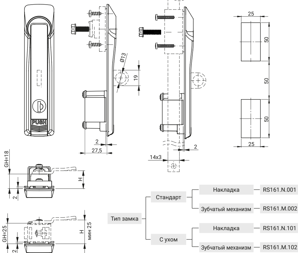
Вид и размер монтажных отверстий
