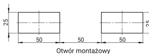
RS150.001SN.M RS150.002SN.M (zamek pod mechanizm zębaty)
