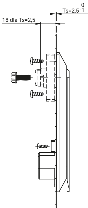
RS150.001SN.N RS150.002SN.N (zamek pod nakładkę)
