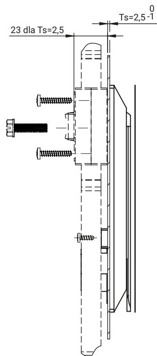
RS150.001SN.M RS150.002SN.M (zamek pod mechanizm zębaty)
