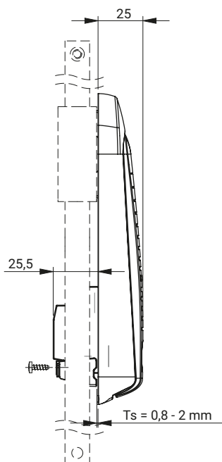
Монтажное отверстие
